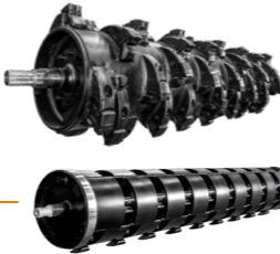
固定ハンマー(UML)または スイングハンマー(FML)付きローター
